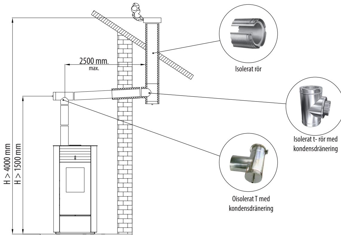
Fig. 9 Rekommenderade längder på delar i kombinerad invändig/utvändig skorsten.
