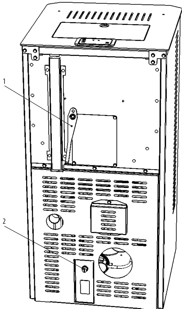
Fig. 19 1. Verktyg för kaminen; 2. Säkerhetstermostat.
