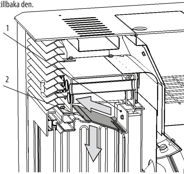
Fig. 16 Borttagning av flamskyddsplåt.
