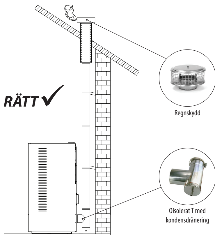
Fig. 6 Hela röckkanalen installerad inne i ett hus.
