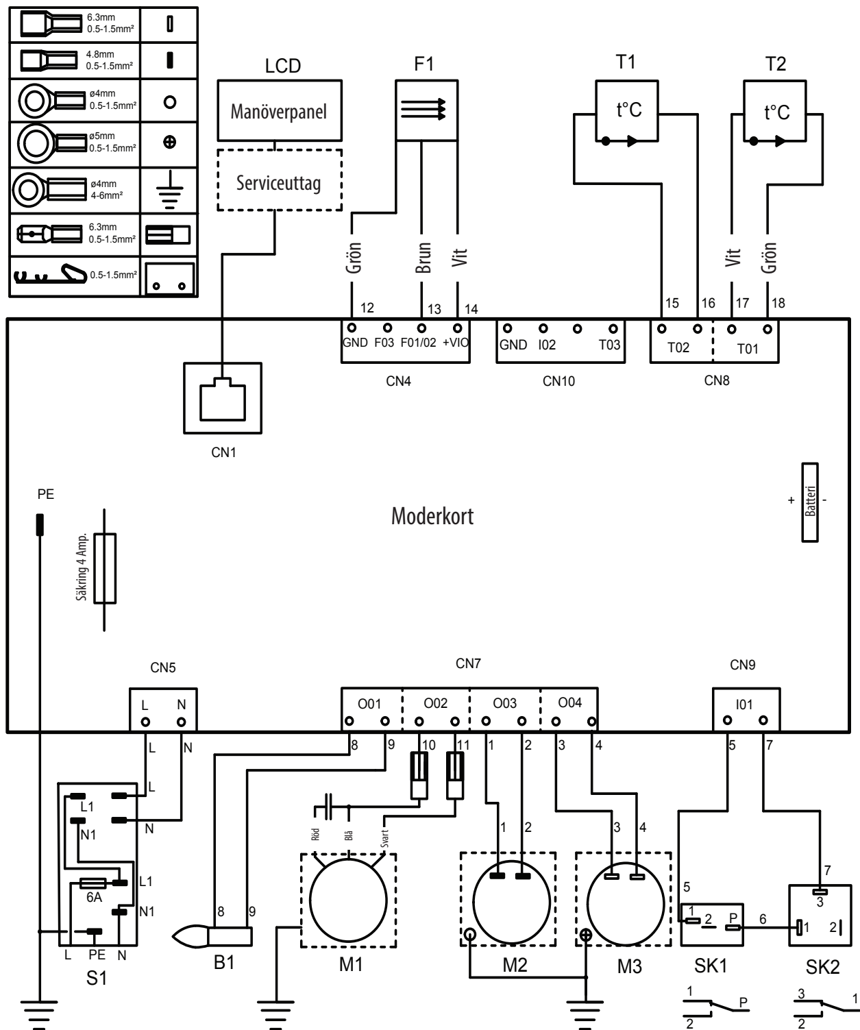
Fig. 2 Kaminens kopplingsschema.
