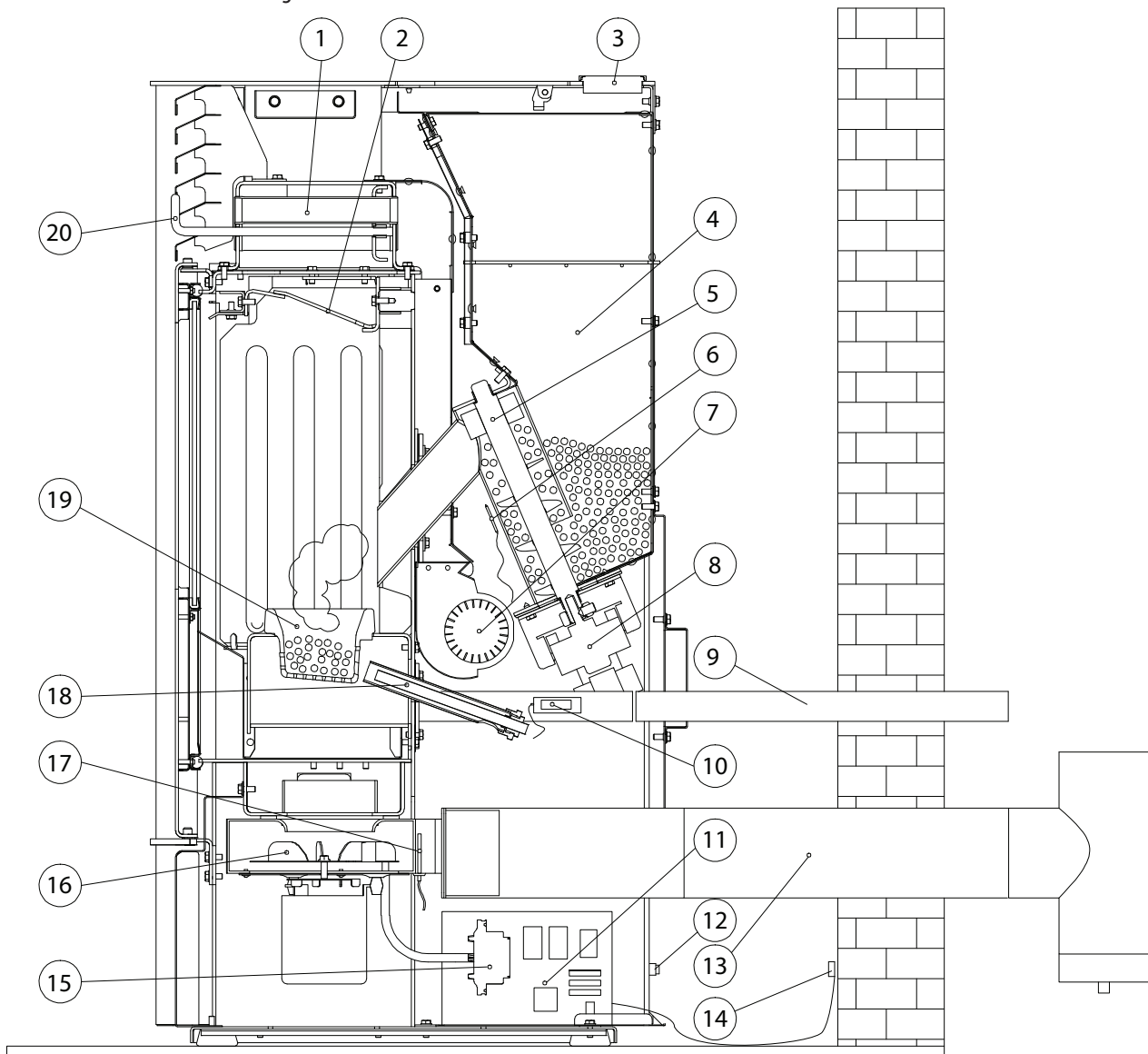
Fig. 1 Komponenter i kaminen
