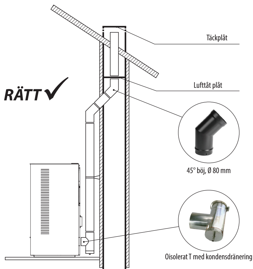
Fig. 5 Rökröret installerat delvis inomhus och delvis i en existerande röckkanal.
