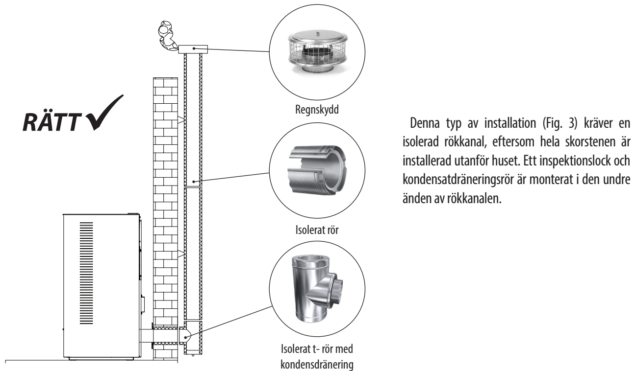
Fig. 3 Skorsten installerad utanför huset.
