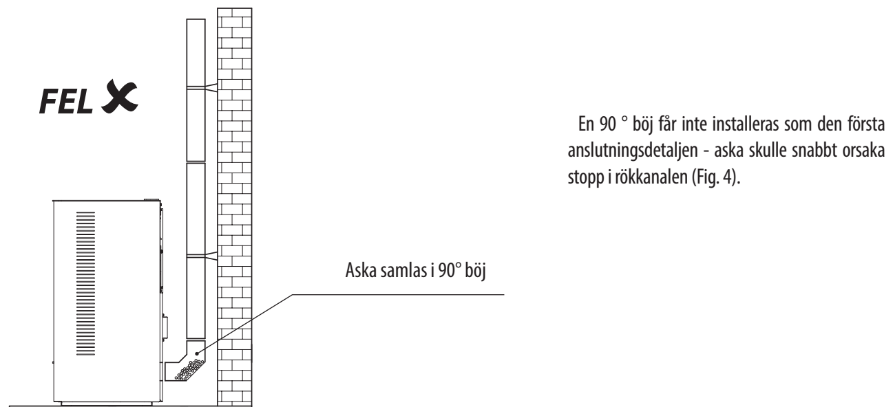
Fig. 4 Felaktig installation - med 90 ° böj som den första anslutningsdetaljen.
