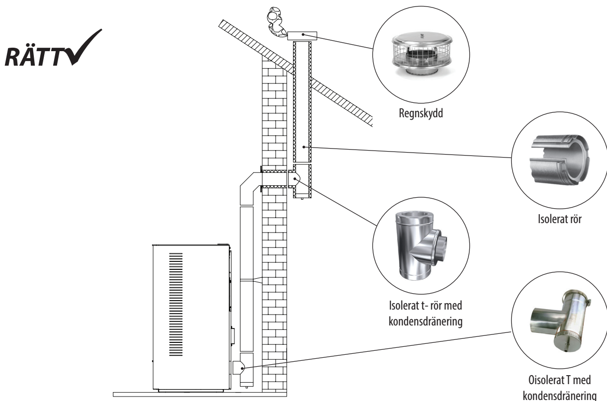
Fig. 8 Installation med en kombinerad intern / extern rökkanal.
