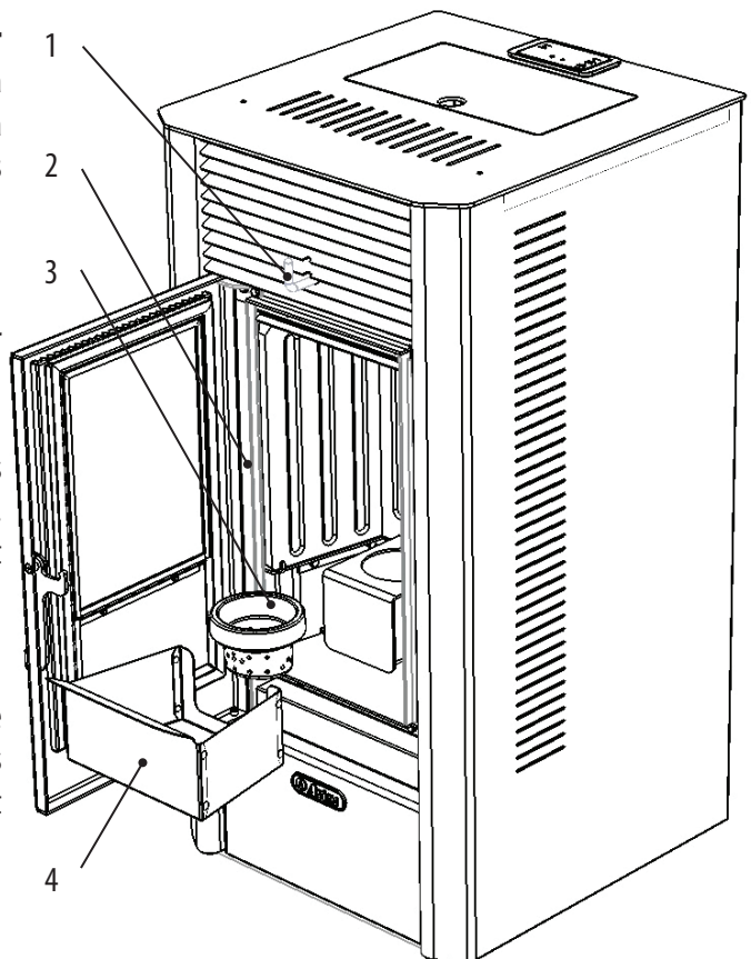
Fig. 12 Delar som behöver kontrolleras ofta och deras plaster.
