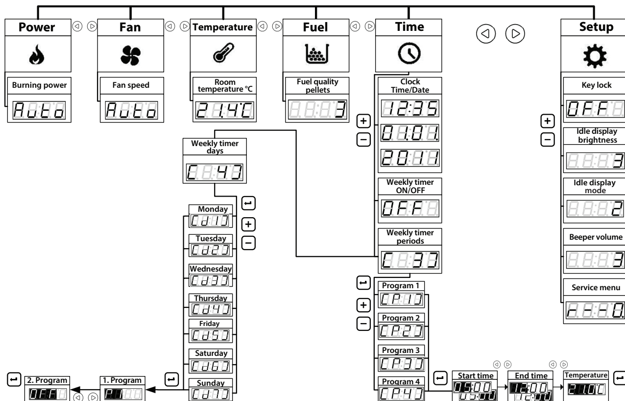
Fig. 11 Menystruktur
