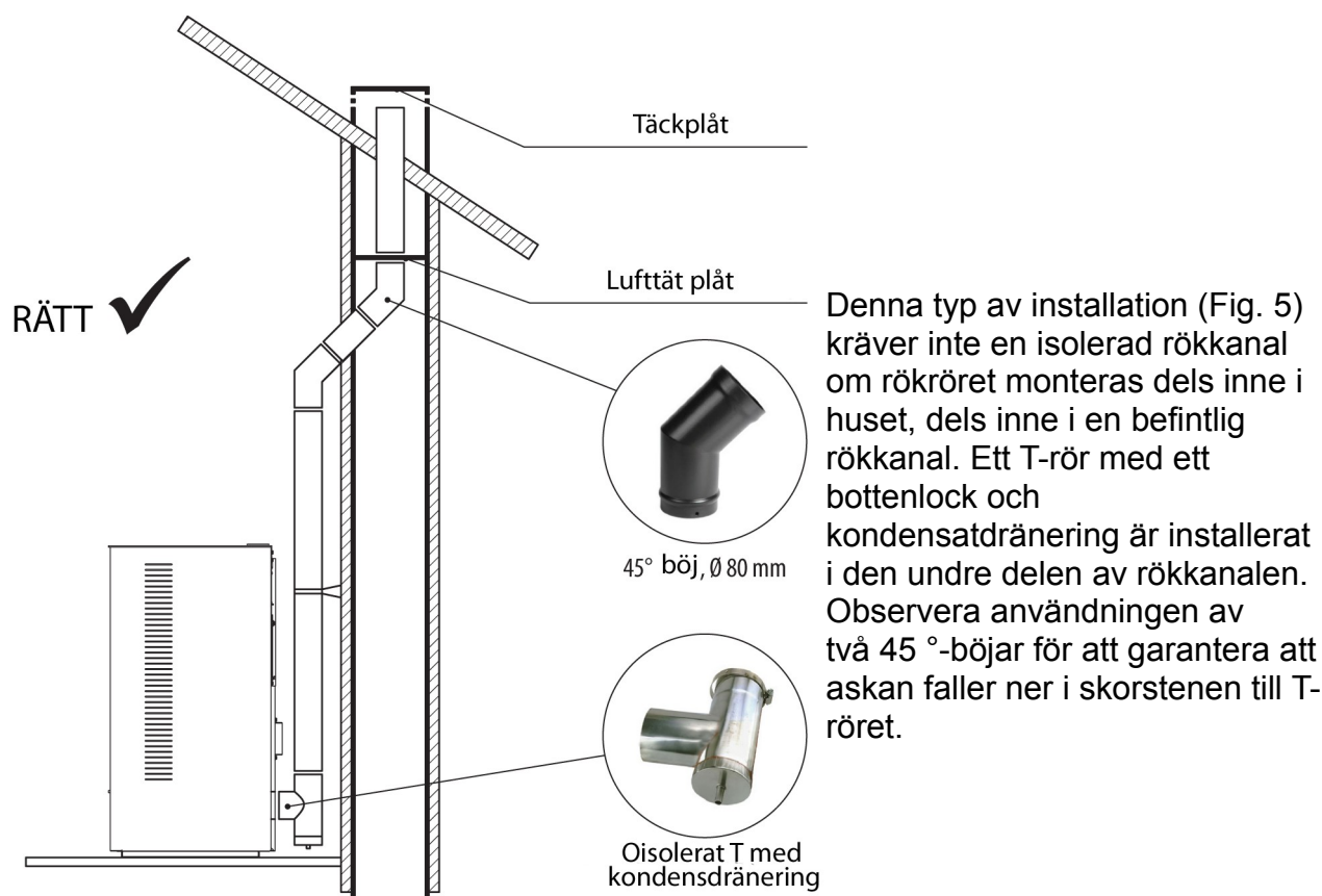
Fig. 5 Rökröret installerat delvis inomhus och delvis i en existerande röckkanal.
