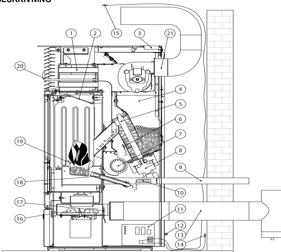
Fig. 1 Komponenter i kaminen
