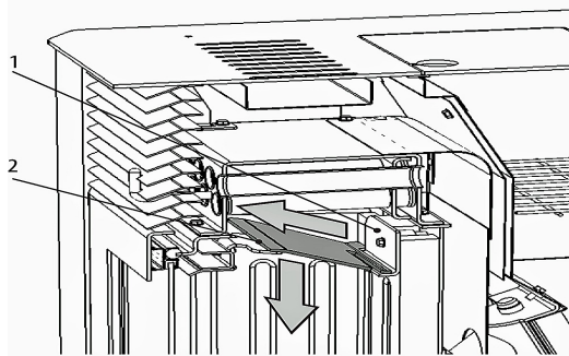
Fig. 16 Borttagning av flamskyddsplåt. 1. Bakre stöd, 2. Främre stöd.
