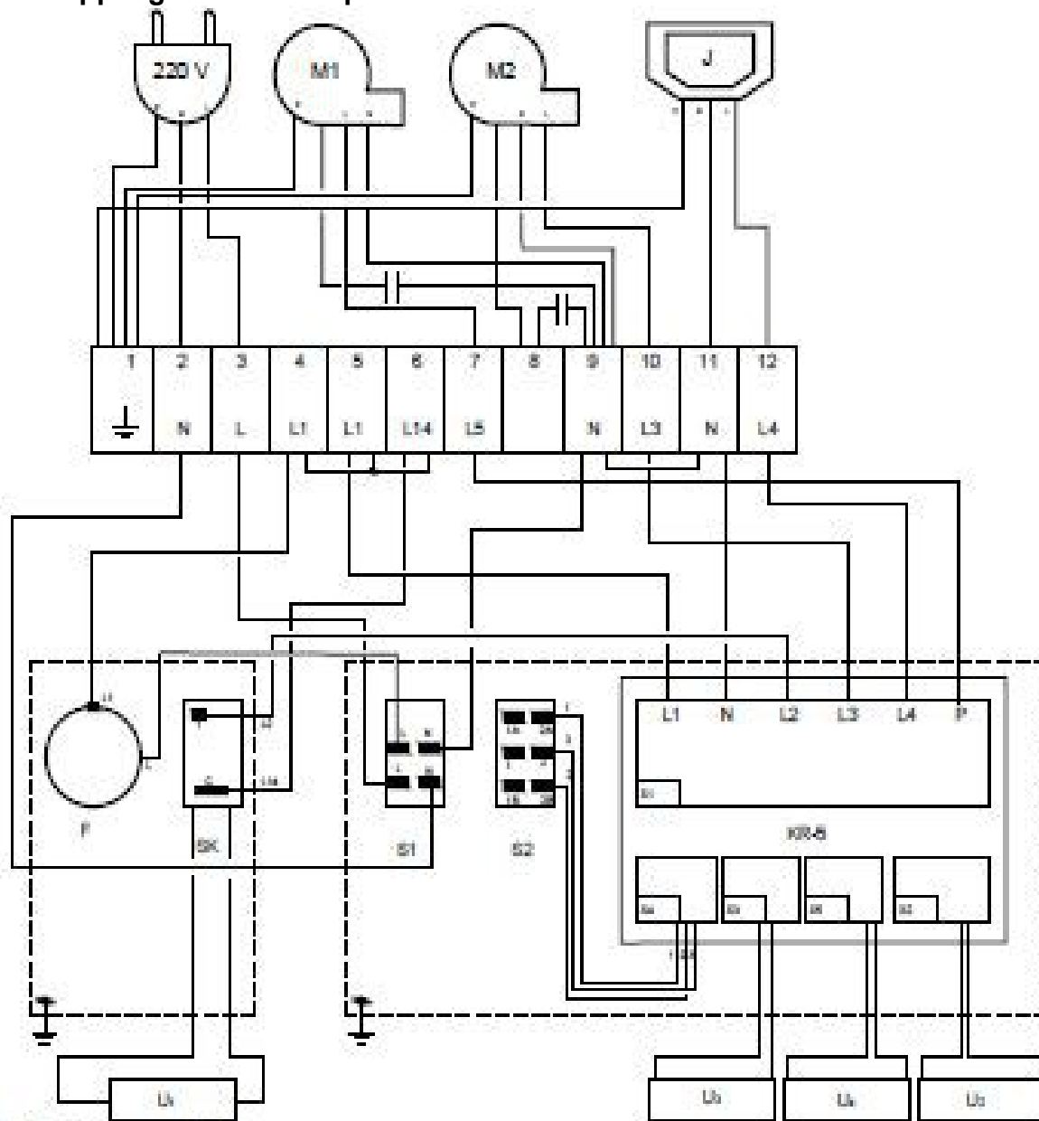
Fig. 6 Kopplingsschema för pannan
