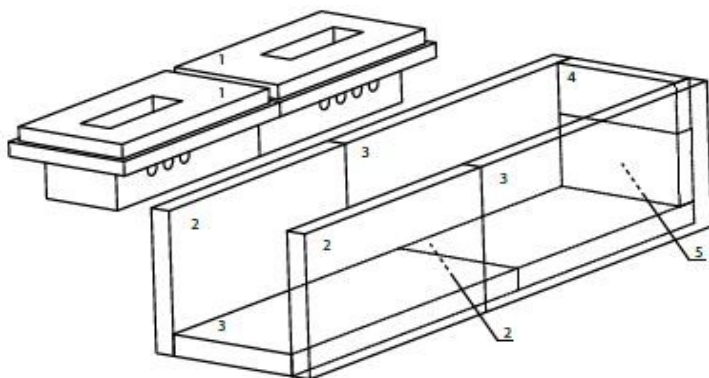
Fig. 2 Keramiska element och deras positioner
