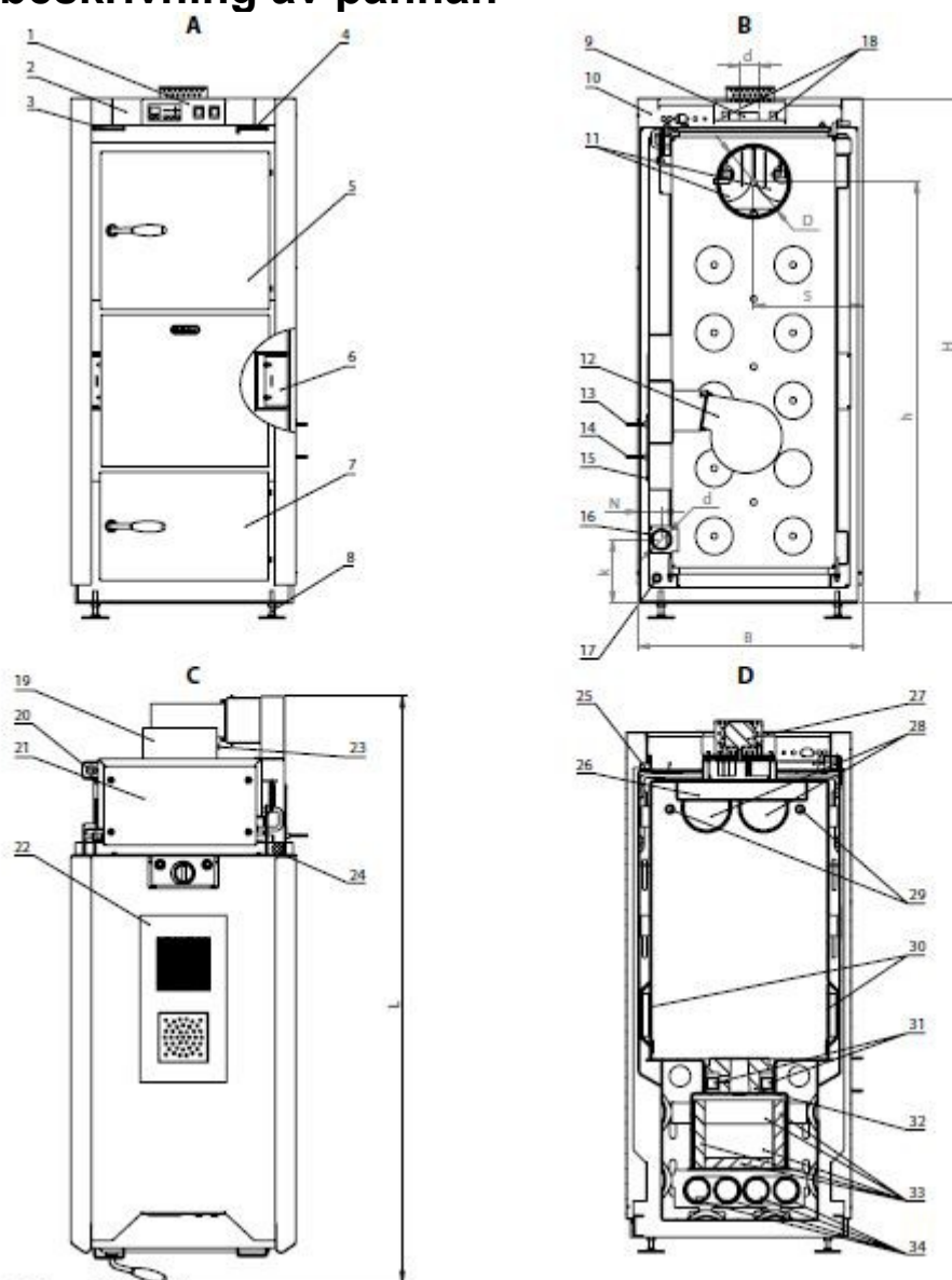
Fig. 1 Allmän överblick över pannan
