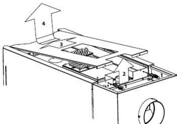
Fig. 7 Demontering av pannans lock
