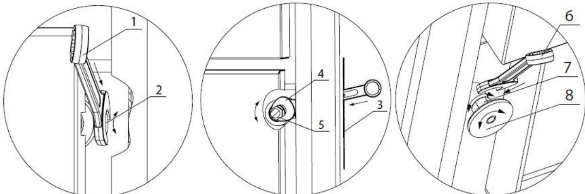
FIG. 13 Justering av luckan och låsmekanismen
