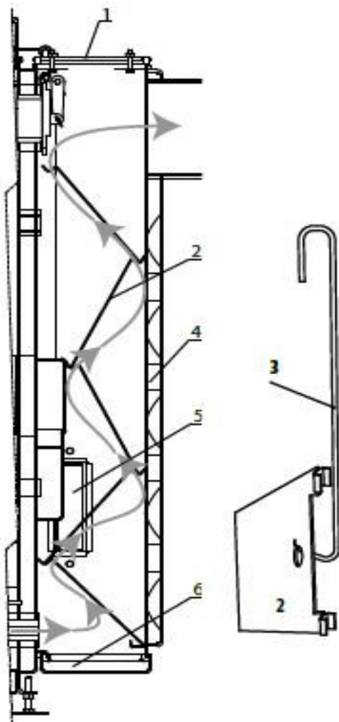
Fig. 3 1. Inspektionslucka, topp, 2. Turbulatorplåtar, 3. Lyftkrok, 4. Värmeväxlare, 5. Inspektionslucka, sida, 6. Inspektionslucka, botten,
