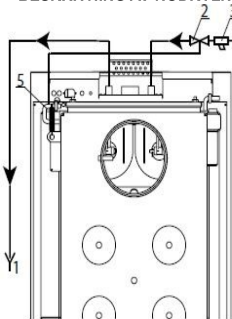
Fig. 4 Kopplingsschema for nödkylsystem
