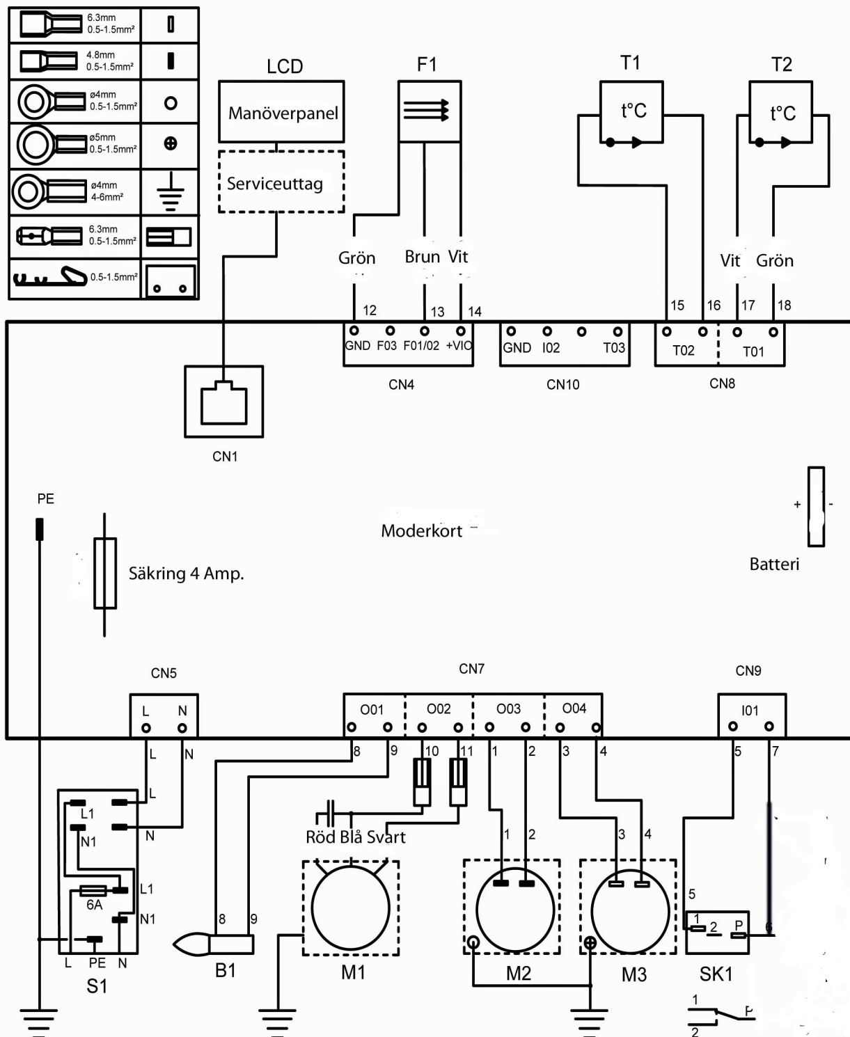
Fig. 2 Kaminens kopplingsschema
