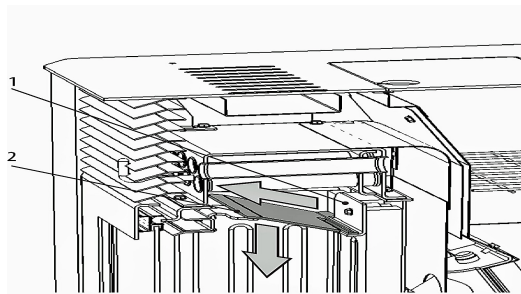
Fig. 16 Borttagning av flamskyddsplåt. 1. Bakre stöd, 2. Främre stöd.
