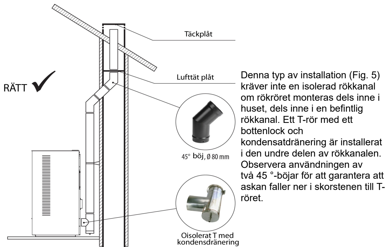
Fig. 5 Rökröret installerat delvis inomhus och delvis i en existerande rökkanal.
