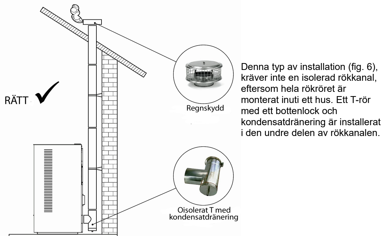
Fig. 6 Hela rökkanalen installerad inne i ett hus.
