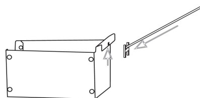
Fig. 20. Verktyg för att lyfta ur het asklåda
