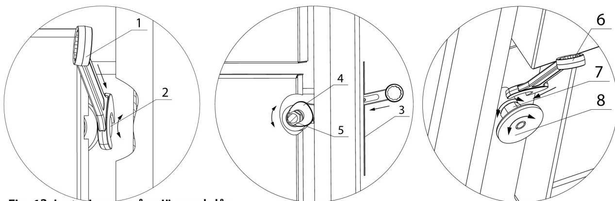
Fig. 13 Justering av gångjärn och lås
