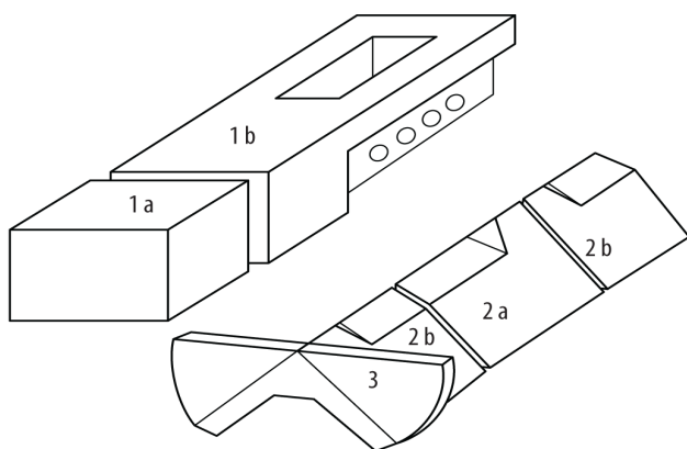
Fig. 2 Keramiska element och deras positioner
