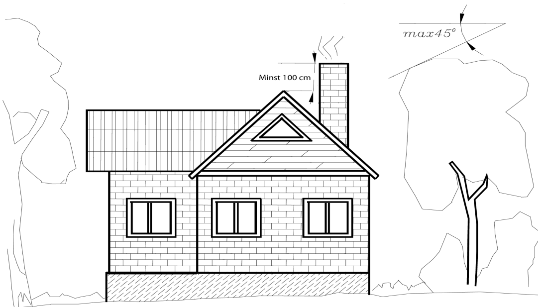
Fig. 8 Höjd på skorstenen i förhållande till omgivningen
