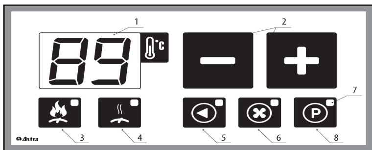
Fig. 11 Frontpanel av regulator KR-4.3D
