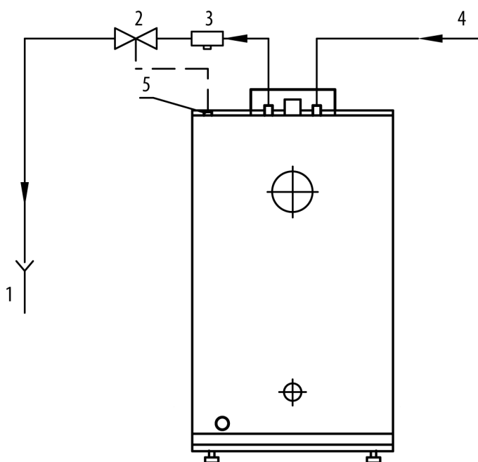
Fig. 4 Kopplingsschema för nödkylsystem
