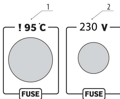
Fig. 10 Bakre kontrollpanel 1. Överhettningsskydd
