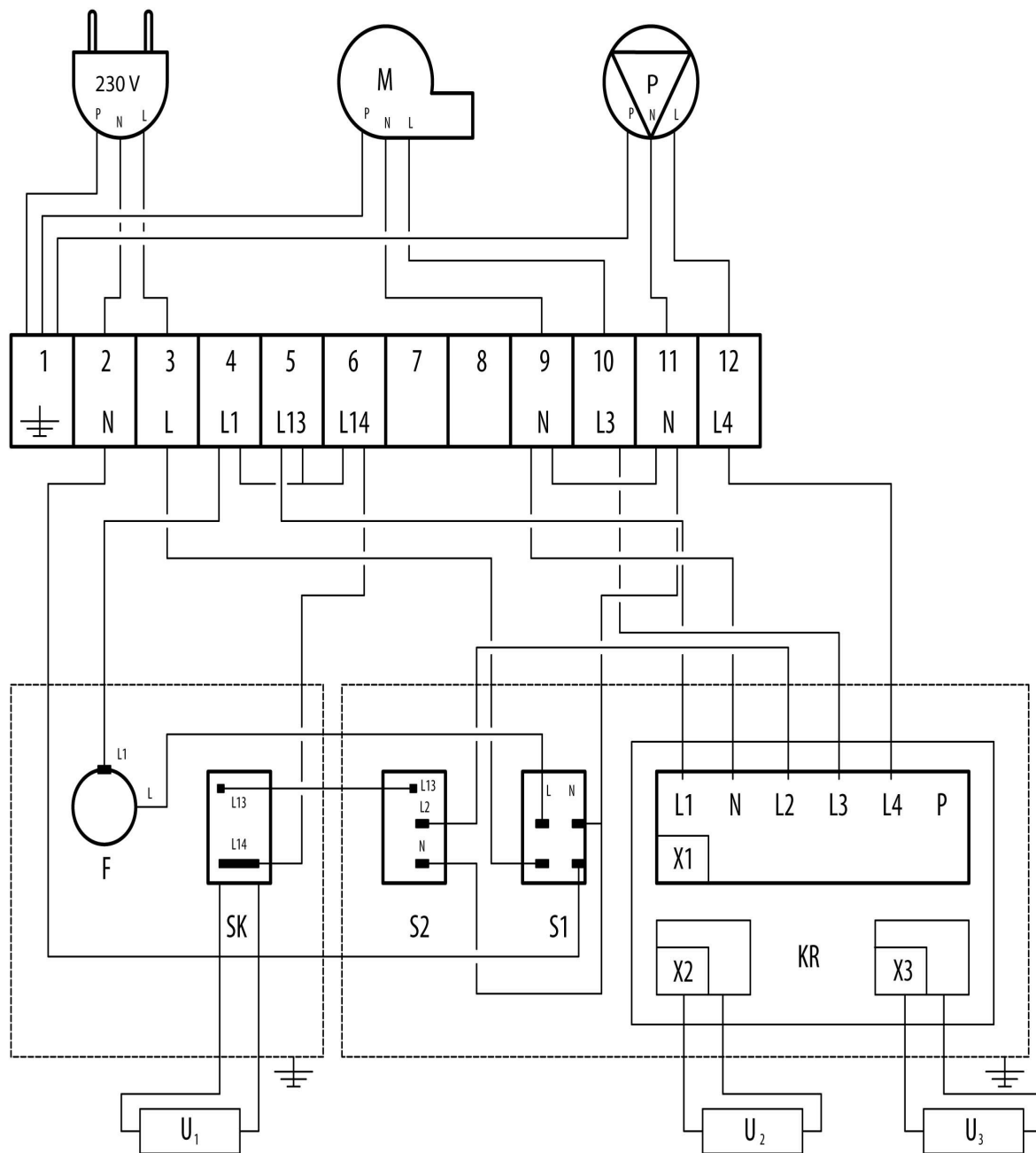
Fig. 6 Kopplingsschema för pannan
