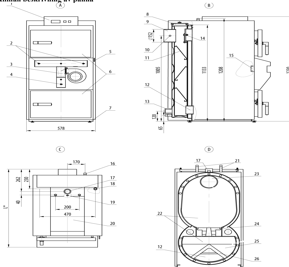
FIG. 1 Allmän överblick över pannan
